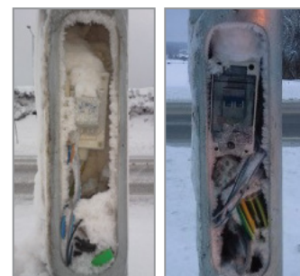
Problemstilling ved installasjon uten vaporplate
