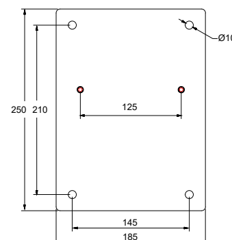
Avlastningsplate for stålfasader eller andre svake fasader
