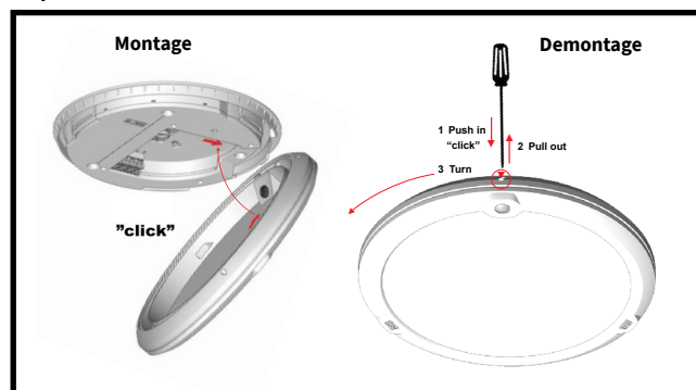
LedgeCircle levereras med bak/sidljus
