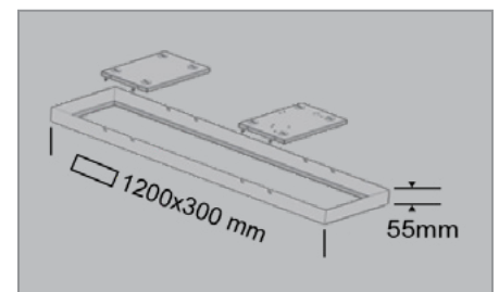
Ramme 1200x300 - utenpåliggende montasje
