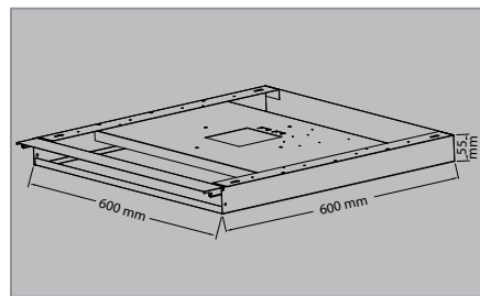
Ramme 600x600 m. luke - utenpåliggende montasje
