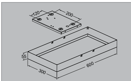
Ramme 600x300 - utenpåliggende montasje
