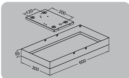
Kehys 600x300 - Pinta-asennus
