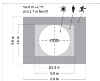
Detekteringsområde for PIR sensor
