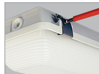
Rustfrie stålklips med sikkerhetsskrue
