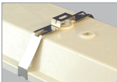
Festebrakett i rustfritt stål - leveres inkl. med armaturen
