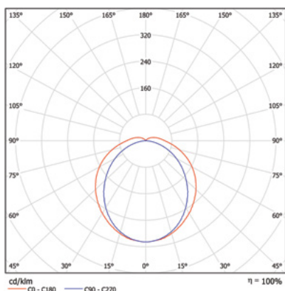
Futurix 37W
