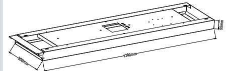
Ramme 1200x300 - luke utenpåliggende montasje
