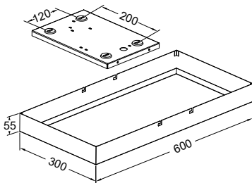
Ramme 300x600 - utenpåliggende montasje
