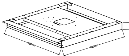
Ramme 600x600 - luke utenpåliggende montasje
