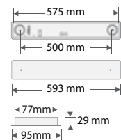
Styringsmodul
